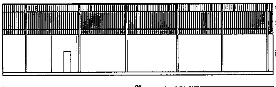
Detalle Elevación H-H' Situación Actual
