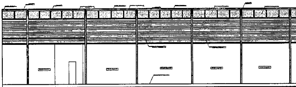
Detalle Elevación H-H' Propuesta
