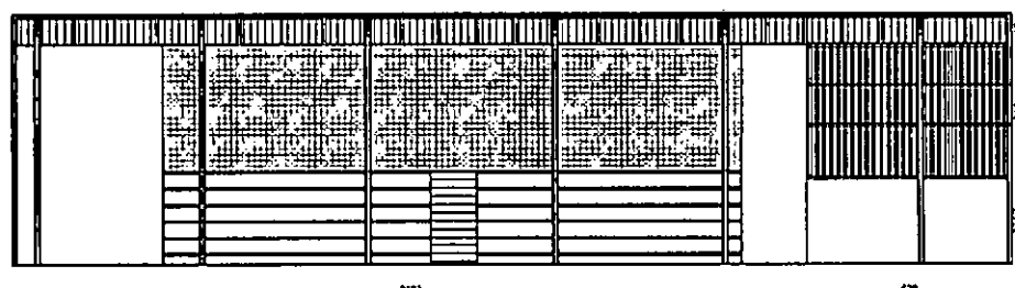
Detalle Elevación I-I' Situación Actual
